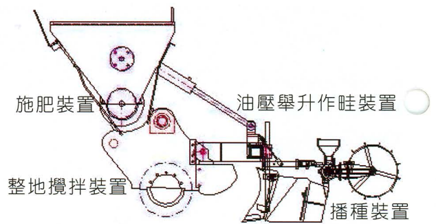
▲圖一、播種施肥作畦一貫作業機示意圖
